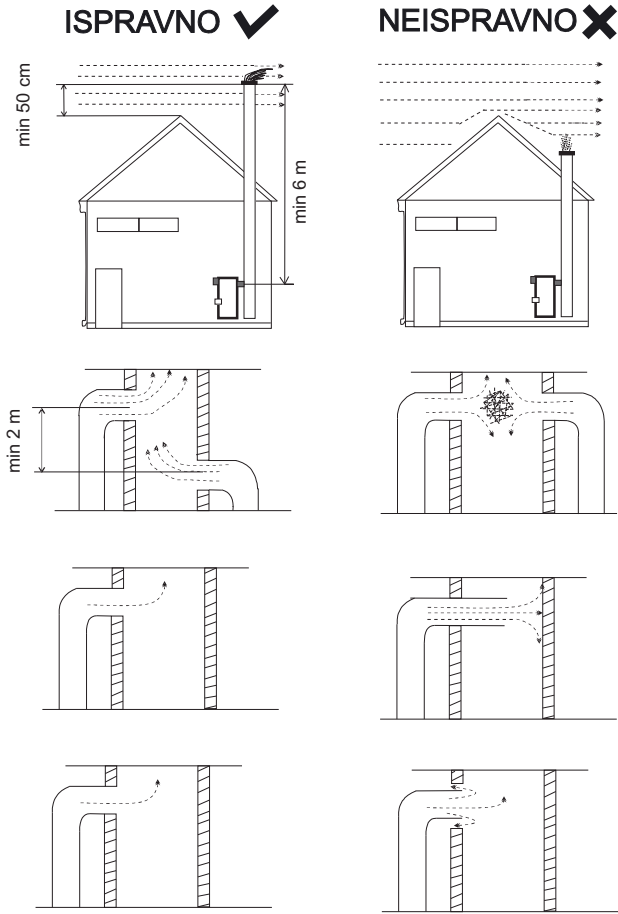
Slika 1. POSTAVLJANJE PEĆI
